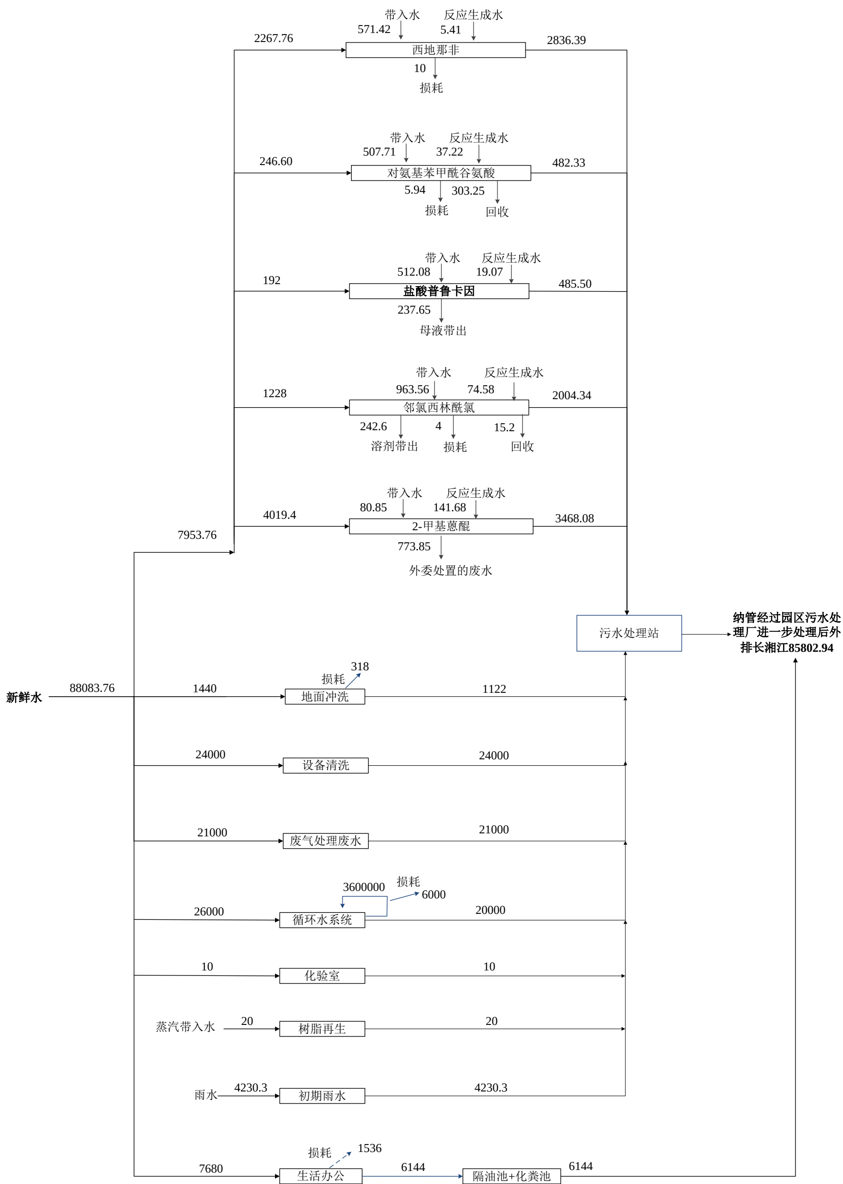
图 4.3-1 变更项目实施后全厂水平衡图 ( \text{m}^3/\text{a} )
