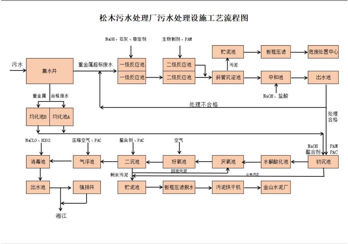
图 8.2-1 松木污水处理厂处理工艺流程图
