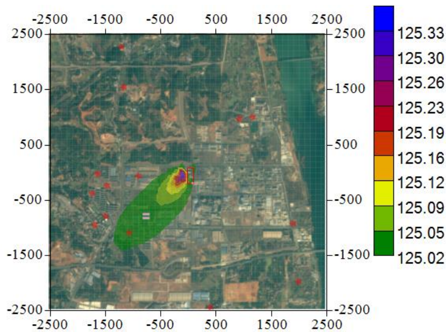
图 7.2.1.7-7 PM_{2.5} 日均浓度叠加在建源污染源及环境质量现状 95%保证率浓度预测结果分布图 ( \mu g/m^3 )
