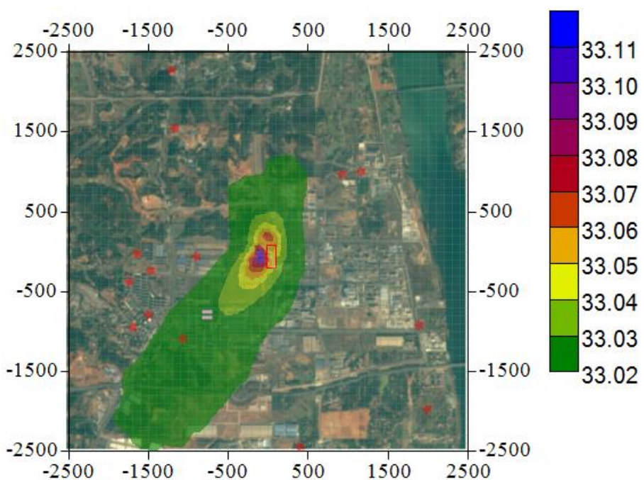
图 7.2.1.7-8 PM_{2.5} 年均浓度叠加在建源及环境质量现状年平均质量浓度预测结果分布图 ( \mu g/m^3 )
