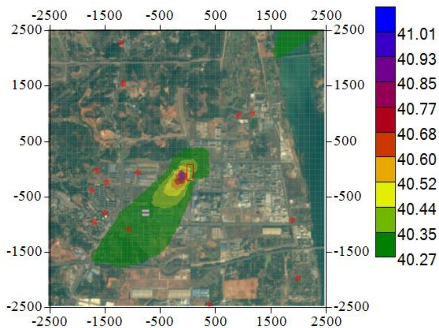
图 7.2.1.7-3 NO 2 日均浓度叠加在建源及环境质量现状 98%保证率浓度预测结果分布图 ( \mu\text{g}/\text{m}^3 )
