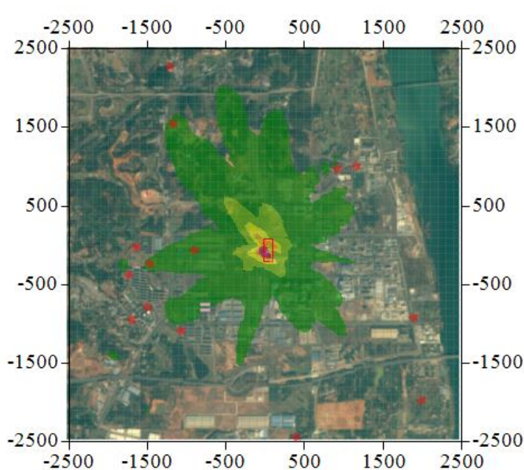
图 7.2.1.7-12 氯小时浓度叠加在建源及环境质量现状浓度预测结果分布图 ( \mu\text{g}/\text{m}^3 )
