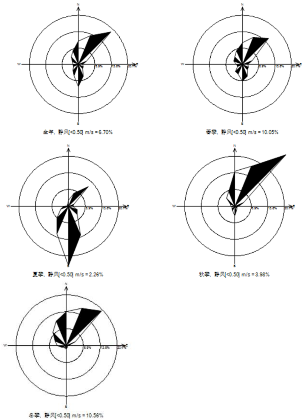
图 7.2.1.4-6 衡阳气象站全年及四季风玫瑰图
