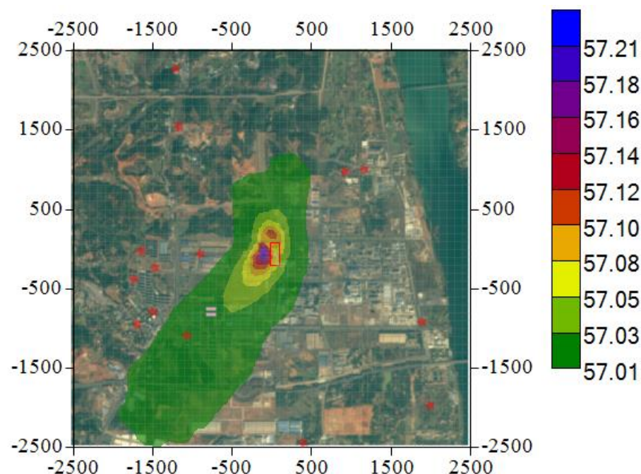
图 7.2.1.7-6 PM_{10} 年均浓度叠加在建源及环境质量现状年平均质量浓度预测结果分布图 ( \mu g/m^3 )
