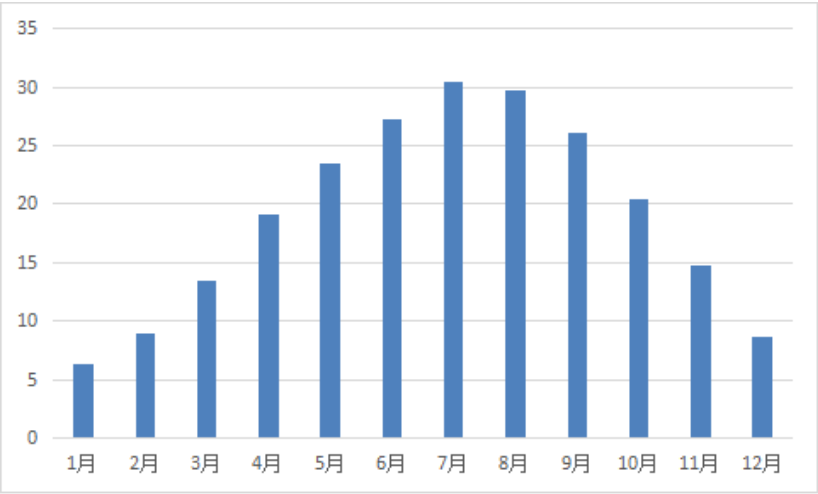
图 7.2.1.4-2 衡阳月平均气温（单位：℃）
