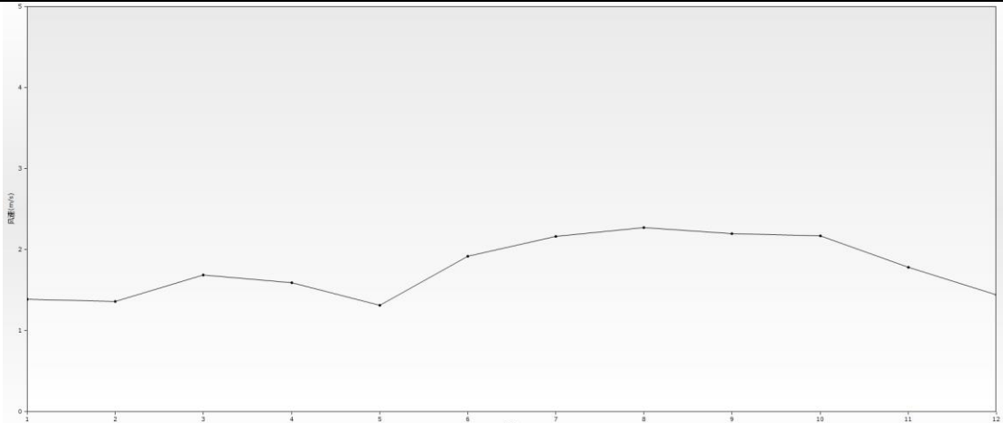
图 7.2.1.4-4 2022 年各月平均风速变化曲线图
