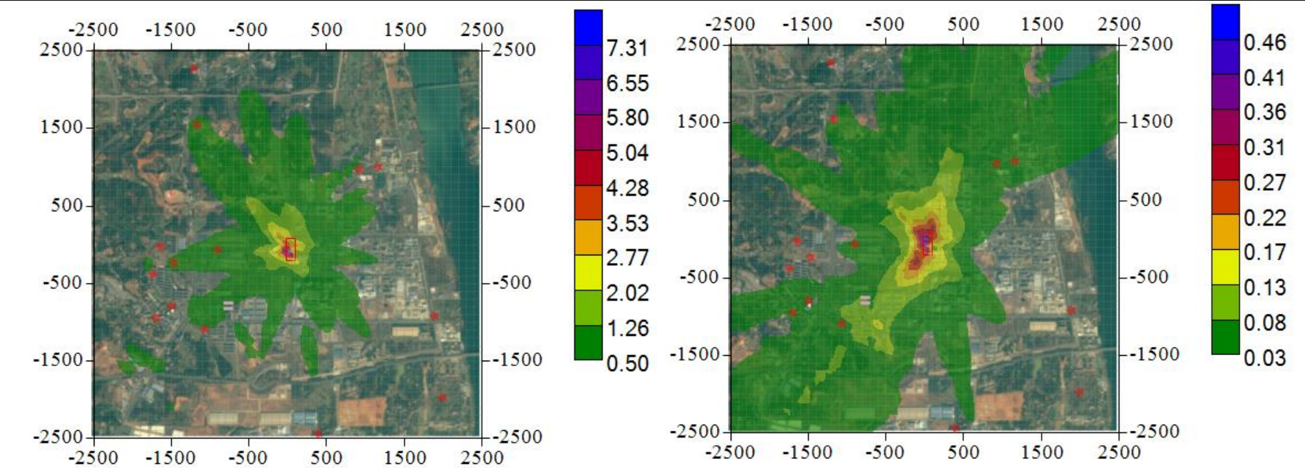
图 7.2.1.7-14 HCl 小时浓度叠加在建源及环境质量现状浓度预测结果分布图（ \mu\text{g}/\text{m}^3 ） 图 7.2.1.7-15 HCl 日均浓度叠加在建源及环境质量现状浓度预测结果分布图（ \mu\text{g}/\text{m}^3 ）
