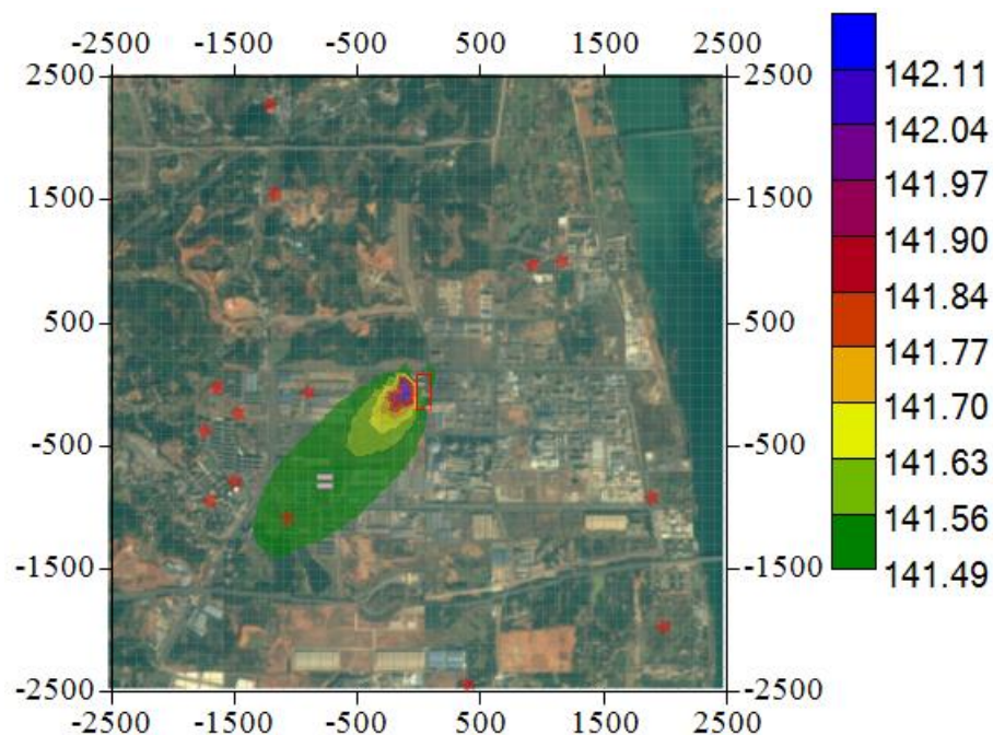
图 7.2.1.7-5 PM_{10} 日均浓度叠加在建源污染源及环境质量现状 95%保证率浓度预测结果分布图 ( \mu g/m^3 )
