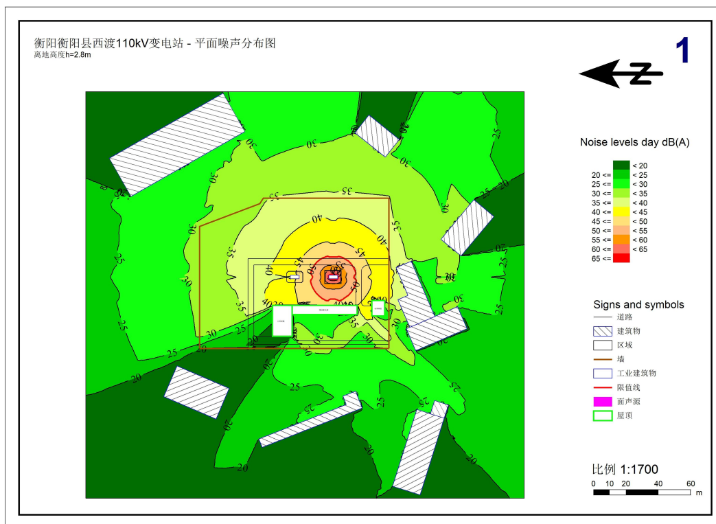
图 4-4 西渡变电站本期规模噪声预测等值线图（围墙上方 0.5m）
