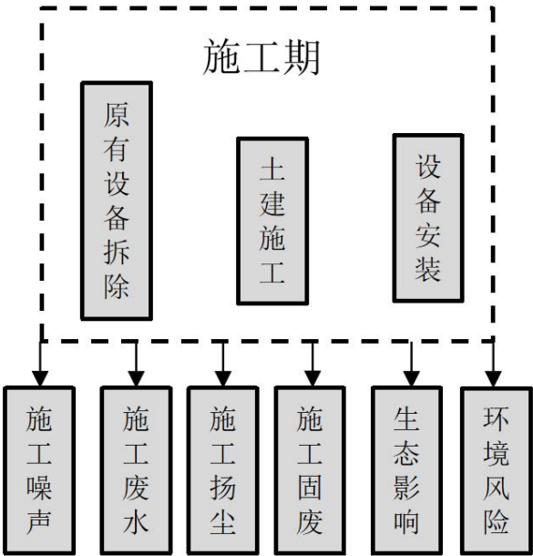
图 4-1 变电站改造工程施工期产污节点图
