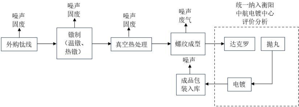
图 2-10 钛合金紧固件工艺流程及产污图
