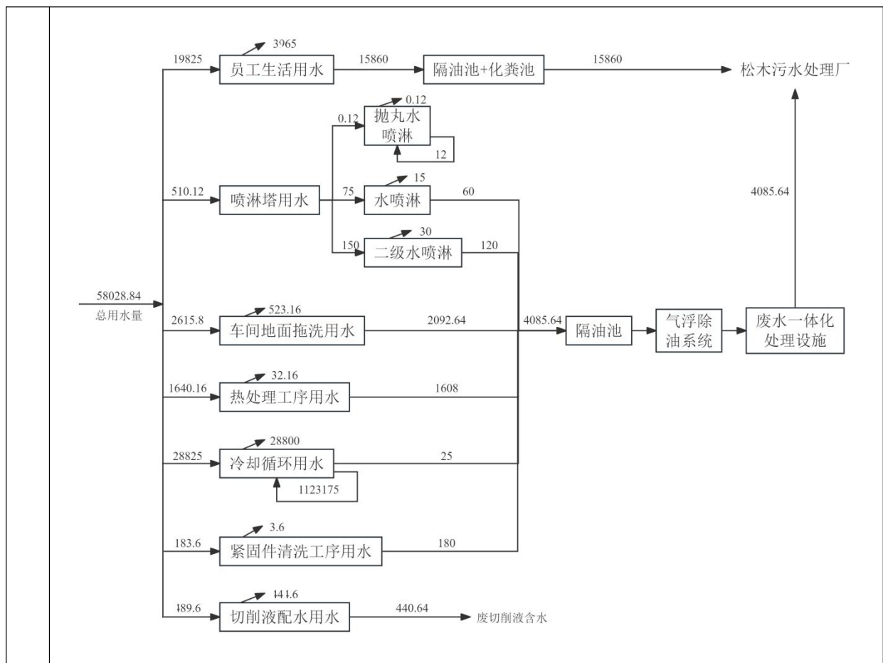
图 2-2 项目建成后全厂水平衡图（m³/a）
